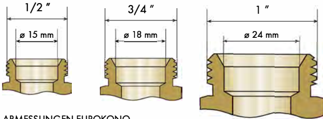
ABMESSUNGEN EUROKONO EUROKONO SIZES
