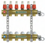
Collectorset messing - 1" V Set collecteur en laiton - 1" F
